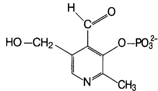
(Пиридоксальфосфат)
