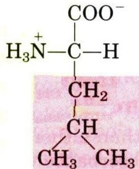
Leucine Лейцин
