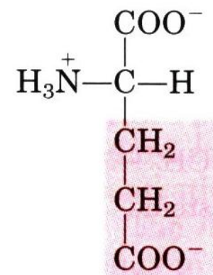
Glutamate Глутамат
