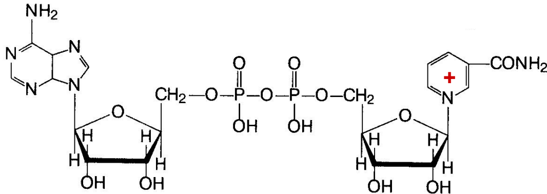
(Н) NAD +
