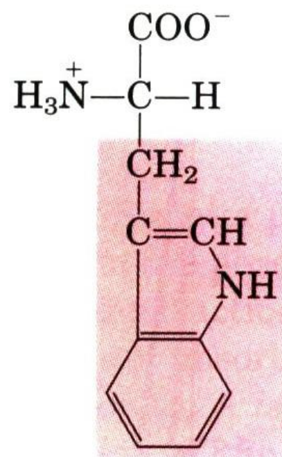
Tryptophan Триптофан
