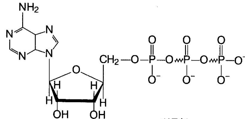
(АТФ)
