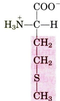
Methionine Метионин
