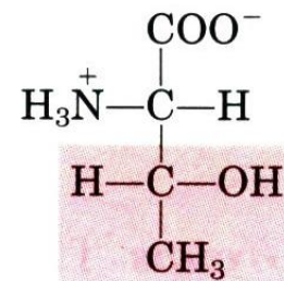
Threonine Треонин
