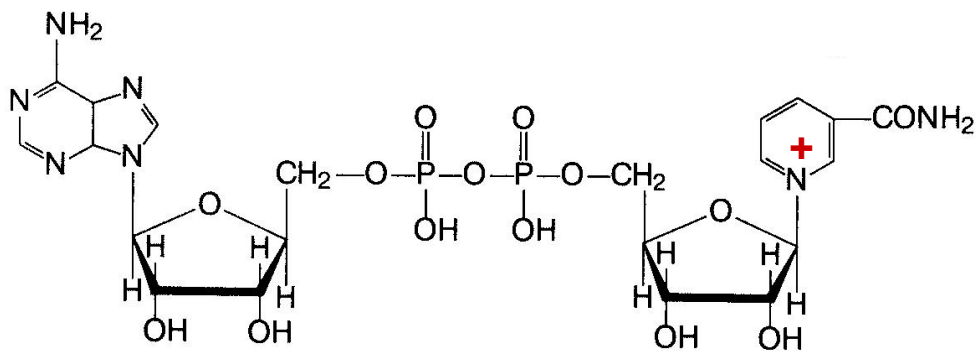
NAD +
