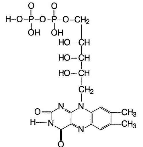
В 2 (Рибофлавинфосфат)
