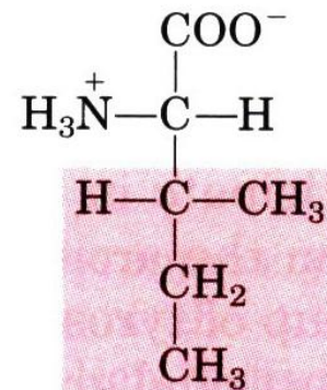
Isoleucine Изолейцин
