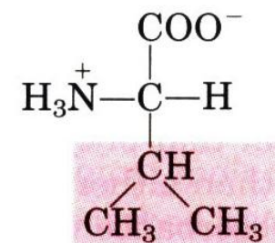
Valine Валин
