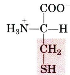
Cysteine Цистеин
