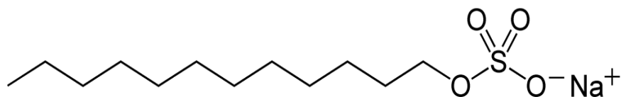
Додецилсульфат натрия
